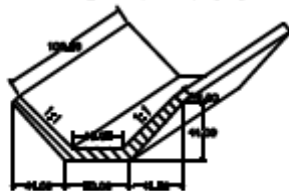
Детайл на отводнителна канавка – готови ст.б. елементи ЕО-1-100
