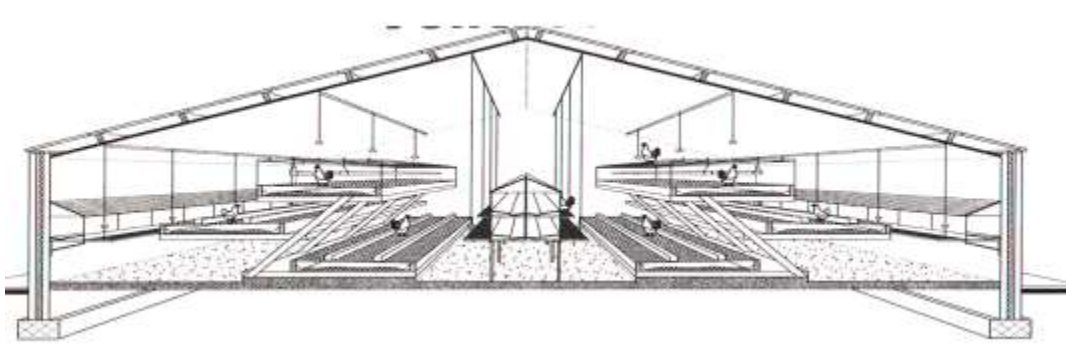
Фиг.1 Волиерна система са отглеждане на кокошки-носачки
